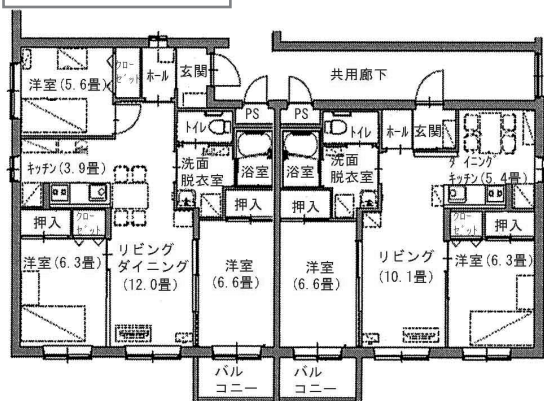
平面詳細図
